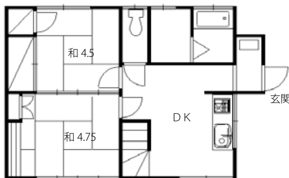
間取図 (略図)
